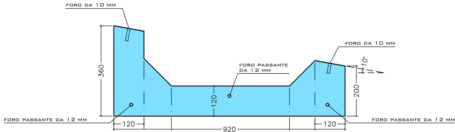
VISTA FRONTALE
