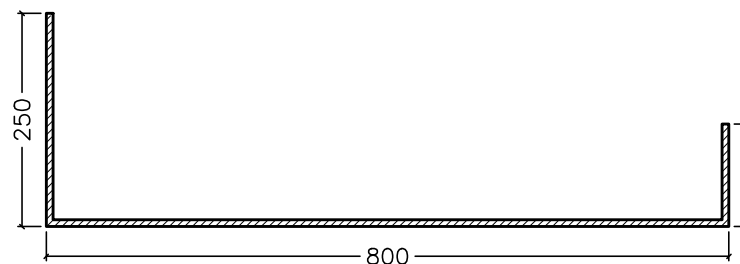
ARMATURA: N. 1 FERRO DA COSTRUZIONE DI DIAMETRO 8 MM
